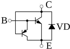
内部等效原理图
