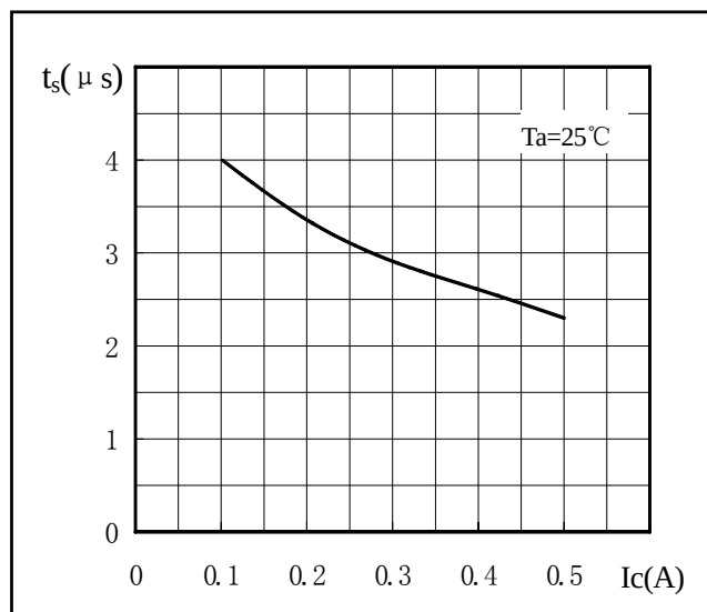
图7 t_s - I_C 关系曲线 (UI9600)
