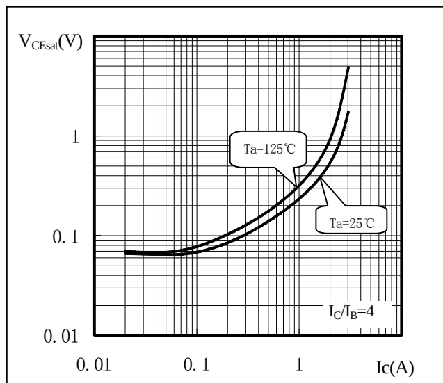
图5 V_{CEsat} - I_C 关系曲线
